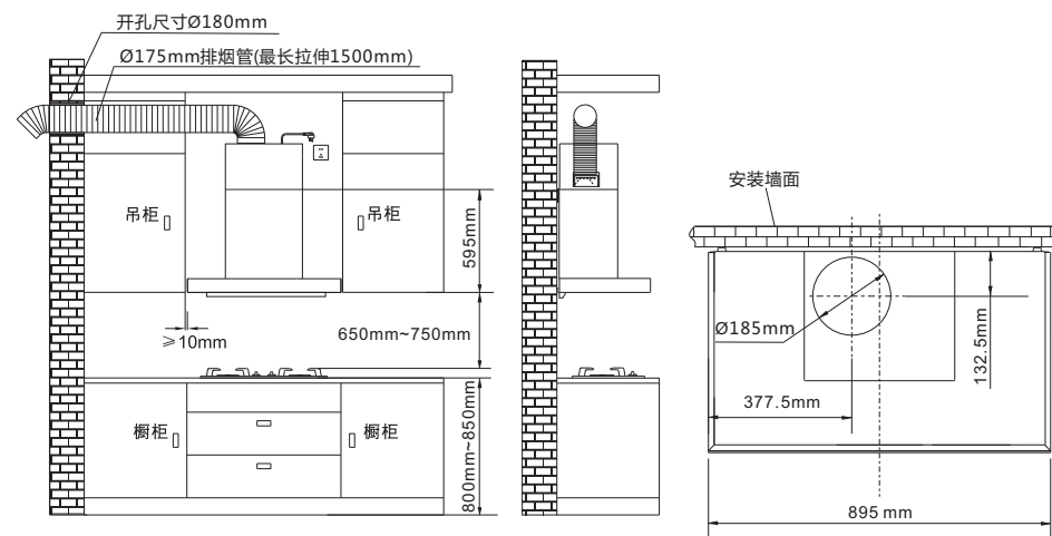
整机与橱柜装配示意图
